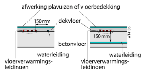
Figuur 19. Minimumafstanden van voorbeeld 5.
