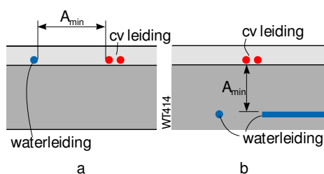
Figuur 11. Minimum afstanden A_{min} tussen waterleiding en cv-leidingen en/of circulatieleidingen voor warmtapwater in tabel 2.
