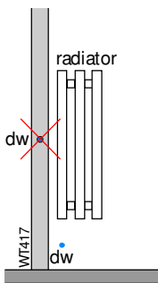
Figuur 15. Waterleiding in wand achter radiator (niet toegestaan)
