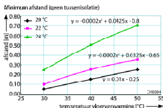
Figuur 20. Interpolatie bij andere aanvoertemperaturen vloerverwarming
