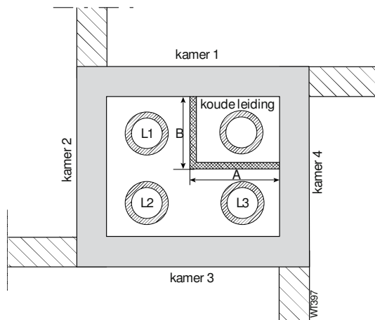
Figuur 7. Doorsnede leidingschacht
