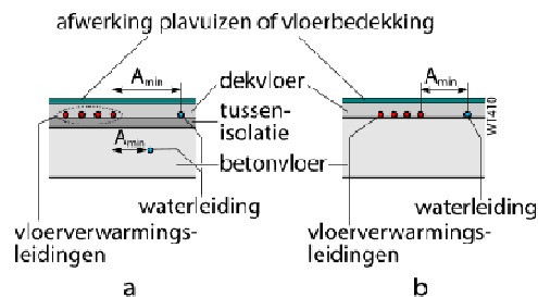
Figuur 17. Minimum afstanden A_{min} vanaf vloerverwarmingsleidingen in tabel 4 en 5
